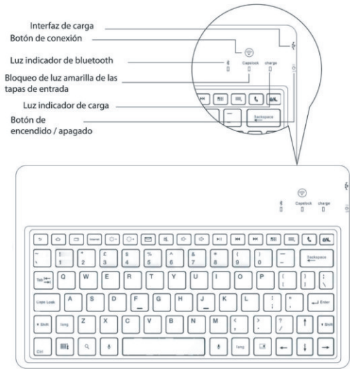
Teclado Bluetooth
